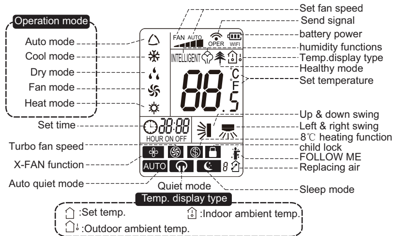
Fig. 3 – Affichage de la télécommande
