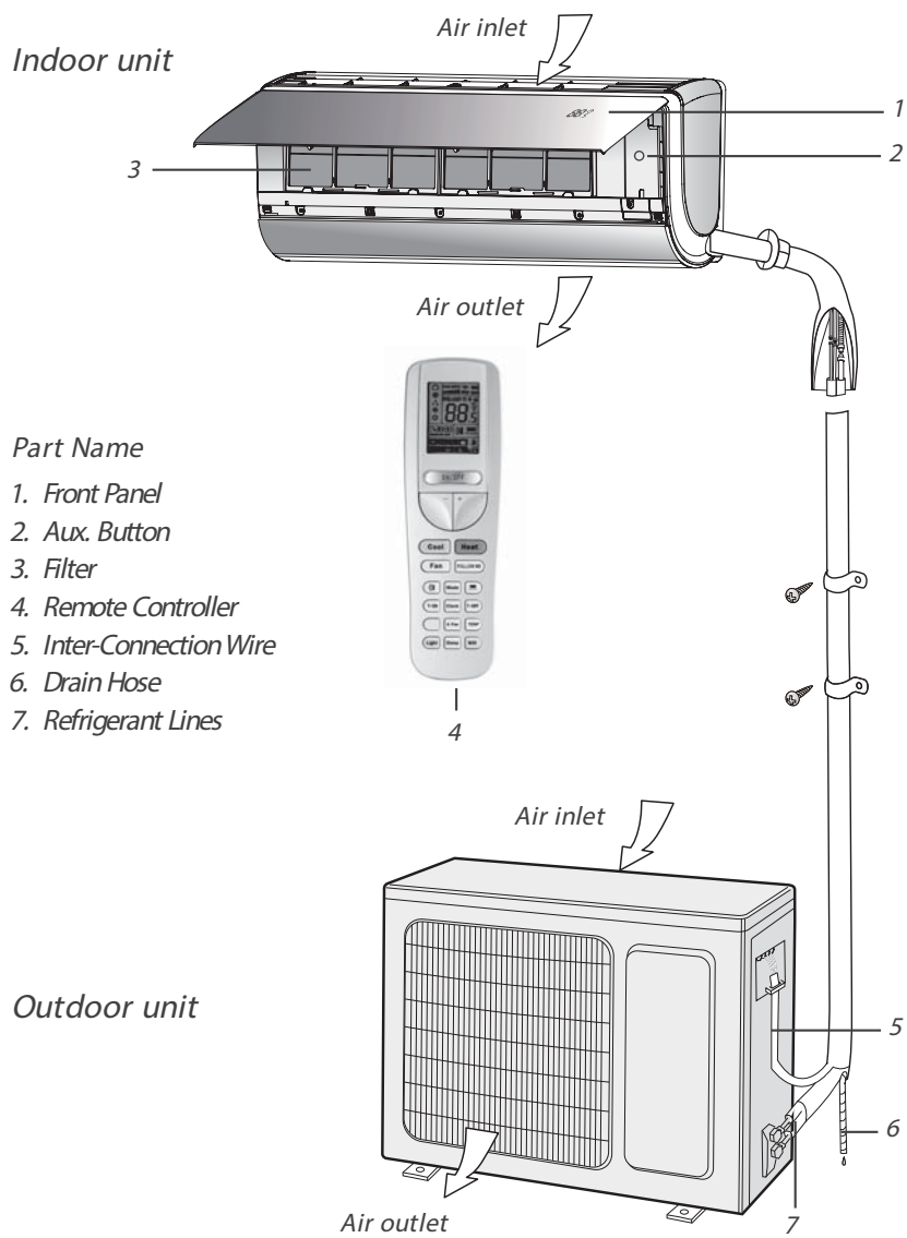
Fig. 1 – Module intérieur/Appareil extérieur
