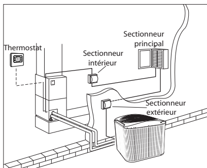
Fig. 1 - Disjoncteurs
